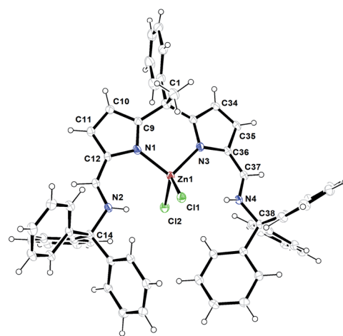
Fig. 2 ORTEP diagram of zinc metal complex ( 4 ) with thermal displacement parameters drawn at the 30% probability level. \text{Zn}1\text{--Cl}1 2.2573(7), \text{Zn}1\text{--Cl}2 2.2301(8), \text{Zn}1\text{--N}1 1.979(2), \text{N}1\text{--C}9 1.347(3), \text{N}1\text{--C}12 1.392(3), \text{C}9\text{--C}10 1.414(4), \text{C}10\text{--C}11 1.366(4), \text{C}11\text{--C}12 1.416(4), \text{C}12\text{--C}13 1.383(4), \text{N}2\text{--C}13 1.347(3), \text{N}2\text{--C}14 1.392(3); \text{N}1\text{--Zn}1\text{--N}3 97.73(9), \text{Cl}1\text{--Zn}1\text{--Cl}2 113.57(3), \text{N}1\text{--Zn}1\text{--Cl}1 112.50(7), \text{N}1\text{--Zn}1\text{--Cl}2 109.54(7), \text{N}3\text{--Zn}1\text{--Cl}1 112.63(7), \text{N}3\text{--Zn}1\text{--Cl}2 109.77(7).
